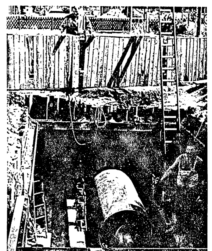
Die Bahn wird durchgepreßt. Unten sieht man des ein Meter dicke Rohr...
