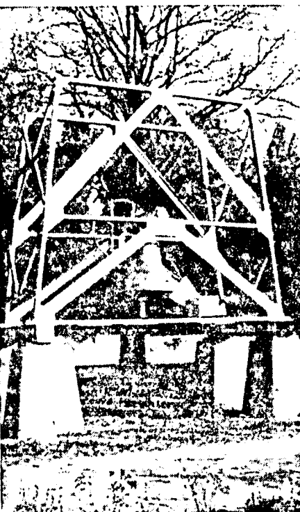
Die Glocke der Petrusgemeinde hängt seit einem Tag in einem Glockenstuhl am Eisensträger, der im Garten vor dem Gemeindeforum in der Bahnhofstraße steht.
