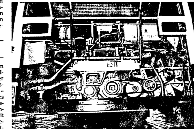
Im Motor des neuen Stadtbusses werden bis zu 90 Prozent der Rußpartikel durch zwei Parallelfilter aufgefangen und danach verbrannt. Foto: kio
