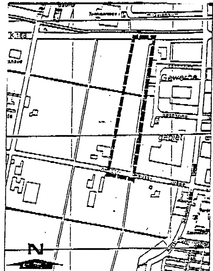
Lageplan (maßstablos) zum Bauleitungsplan H 05/01 „An der Knappeswiese“
